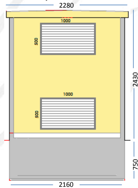
FAÇADE GAUCHE
