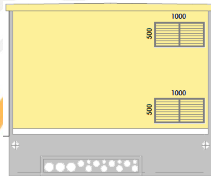
FAÇADE GAUCHE
